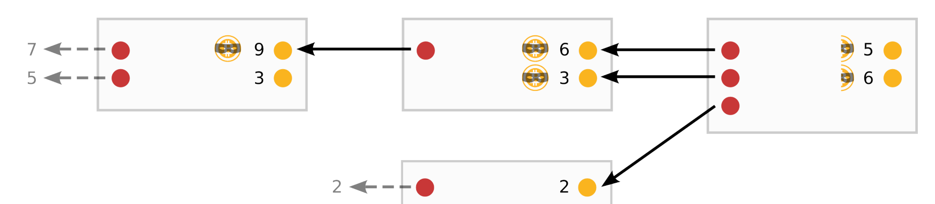
Abb. 9: Umsetzung der anteiligen Vergiftung, Darstellung analog zu Abb. 4, ● gesperrte Transaktionsausgänge, ● anteilig gesperrte Transaktionsausgänge
