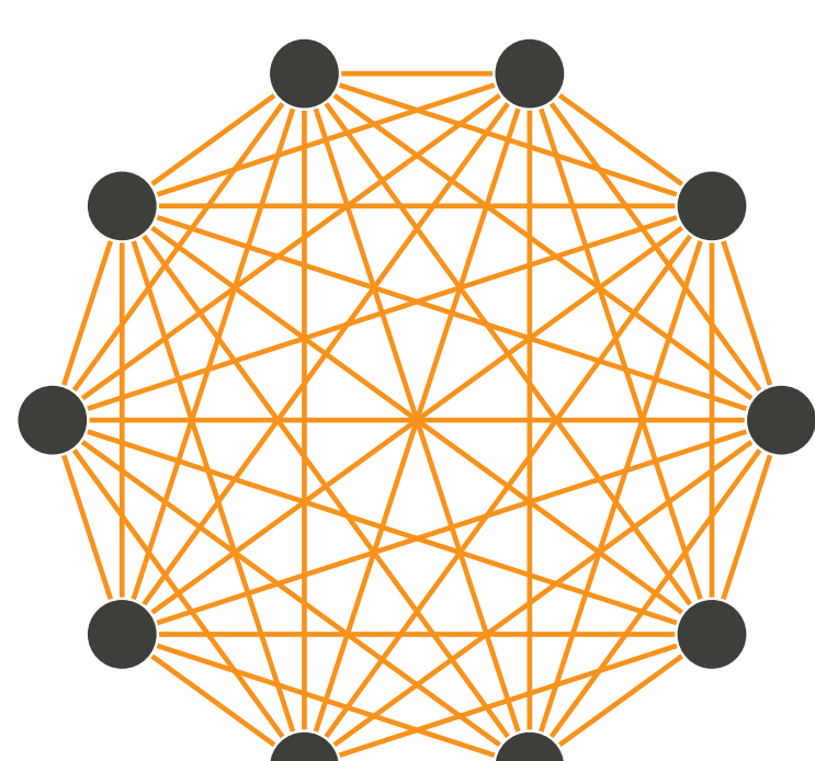
Abb. 3: P2P-Netzwerk
